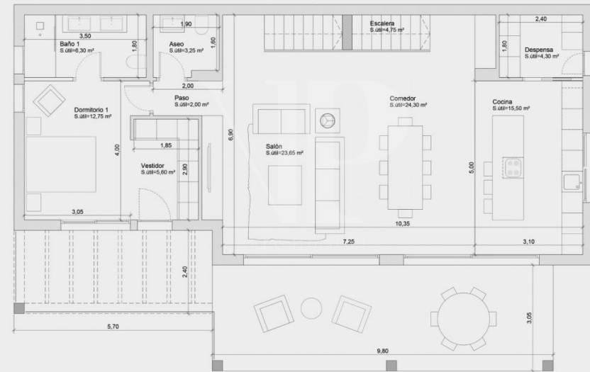
PLANTA BAJA Sup. construida vivienda 119,17 m 2 Sup. construida porche 29,90 m 2
