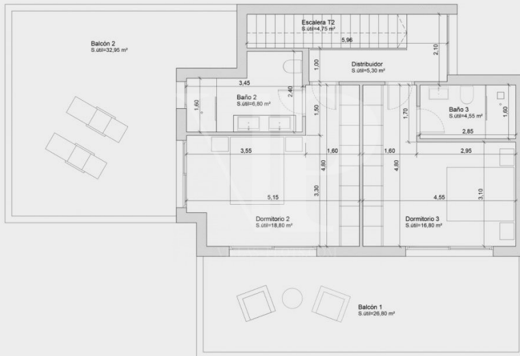
PLANTA PRIMERA Sup. construida vivienda 69,70 m²
