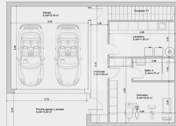
PLANTA SÓTANO Sup. construida vivienda 95,43 m 2 Sup. construida porche 13,68 m 2
