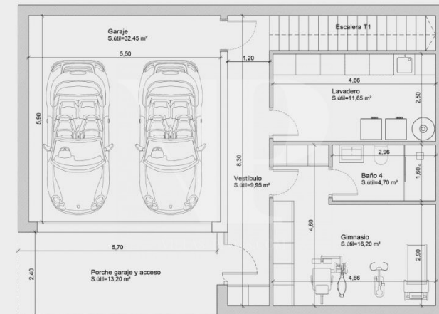
PLANTA SÓTANO Sup. construida vivienda 95,43 m² Sup. construida porche 13,68 m²
