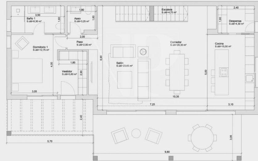
PLANTA BAJA Sup. construida vivienda 119,17 m² Sup. construida porche 29,90 m²
