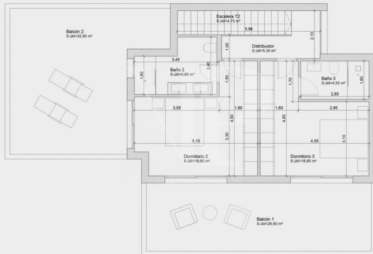
PLANTA PRIMERA Sup. construida vivienda 69,70 m 2
